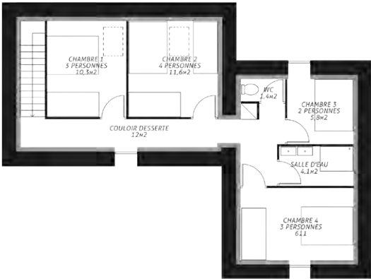
Plan ETAGE 1 ech 1/75 - sous réserve relevé précis
