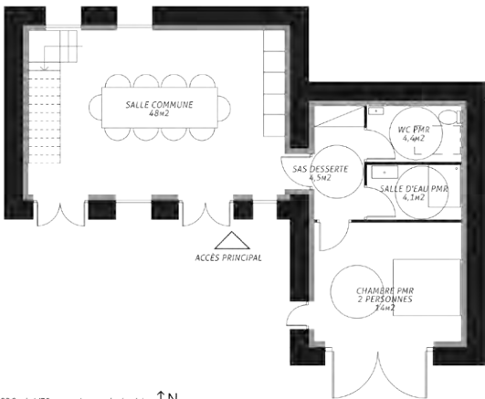
Plan RDC ech 1/75 - sous réserve relevé précis
