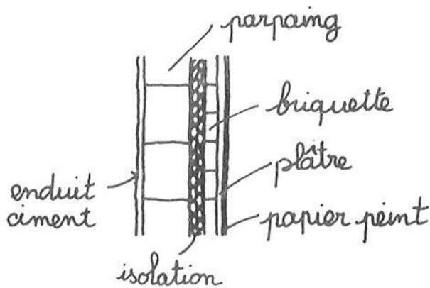
Coupe d'un mur
