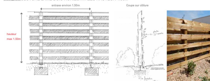
TYPE 1 : CLÔTURE LAME BOIS HORIZONTALES HAUTEUR 1.50M
